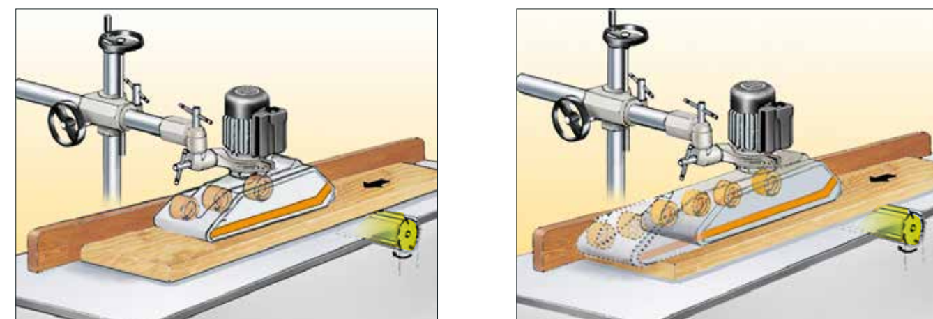
PIALLA A FILO / THICKNESSER PLANER / DEGAUCHISSEUSE / CEPILLADORA
